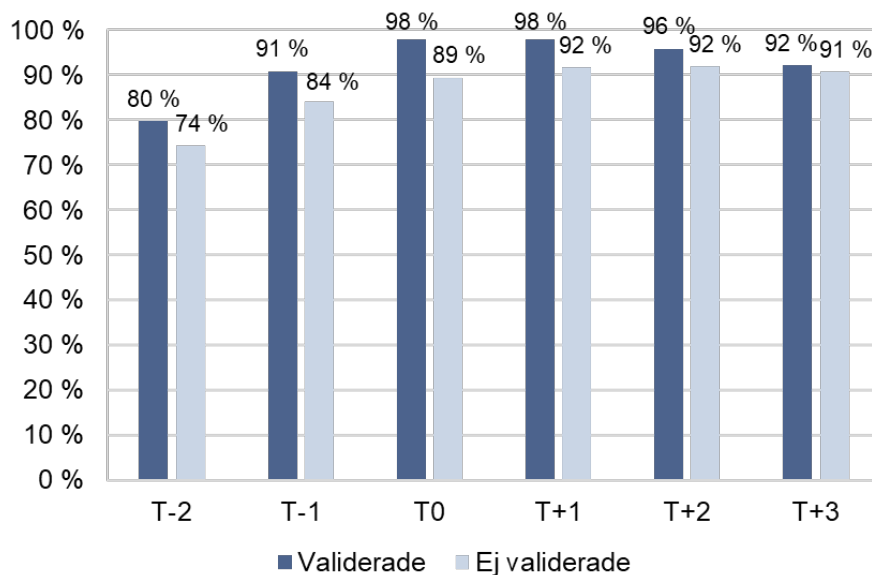
Diagram 5. Andel i arbete, validerade och ej validerade, från två år innan avslut till tre år efter avslut.
