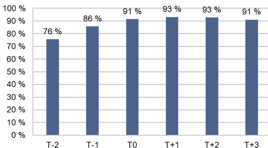
Diagram 4. Andel i arbete, från två år innan avslut till tre år efter avslut.
