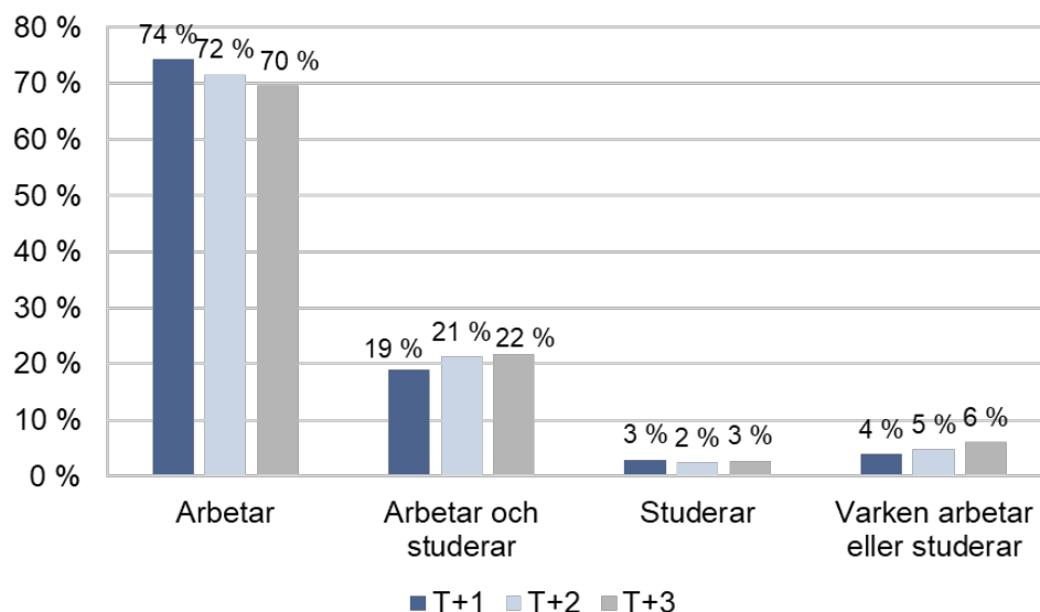
Diagram 6. Kategoriserad sysselsättning, ett till tre år efter avslut.
