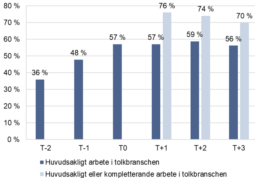
Diagram 8. Arbete inom tolkbranschen, två år innan avslut till tre år efter avslut. Avser de i arbete under det aktuella året.
