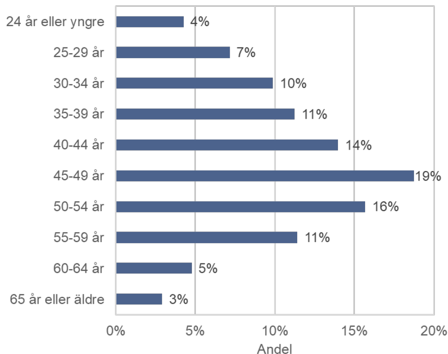
Diagram 2. Åldersfördelning bland deltagarna.
