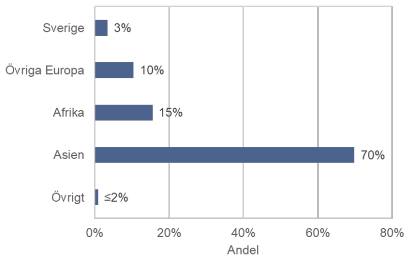
Diagram 3. Födelsevärldsdel bland deltagarna.
