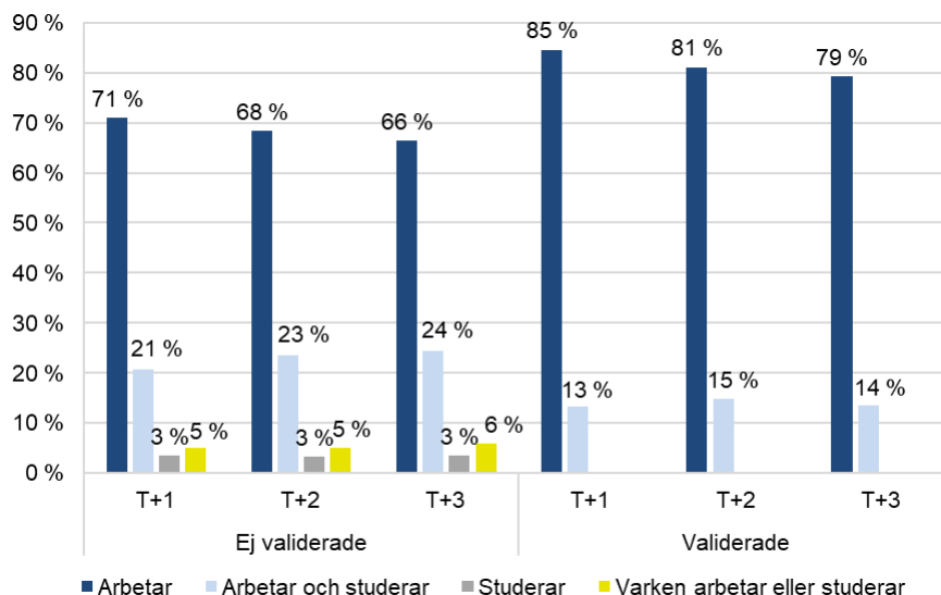
Diagram 7. Kategoriserad sysselsättning, validerade och ej validerade, ett till tre år efter avslut.
