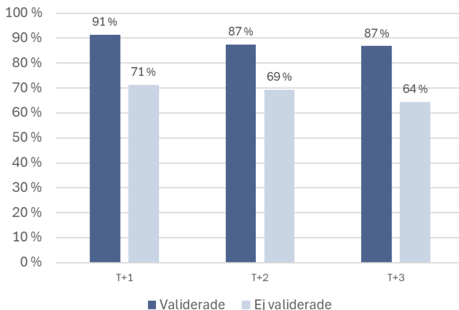
Diagram 10. Arbete (huvudsakligt eller kompletterande arbete) inom tolkbranschen, efter validerade och ej validerade, ett till tre år efter avslut. Avser de i arbete under det aktuella året.
