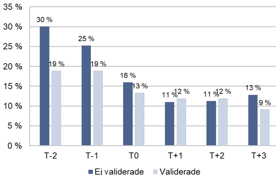
Diagram 12. Andel deltagare med registrerad arbetslöshet (validerade och ej validerade), från två år innan avslut till tre år efter avslut.
