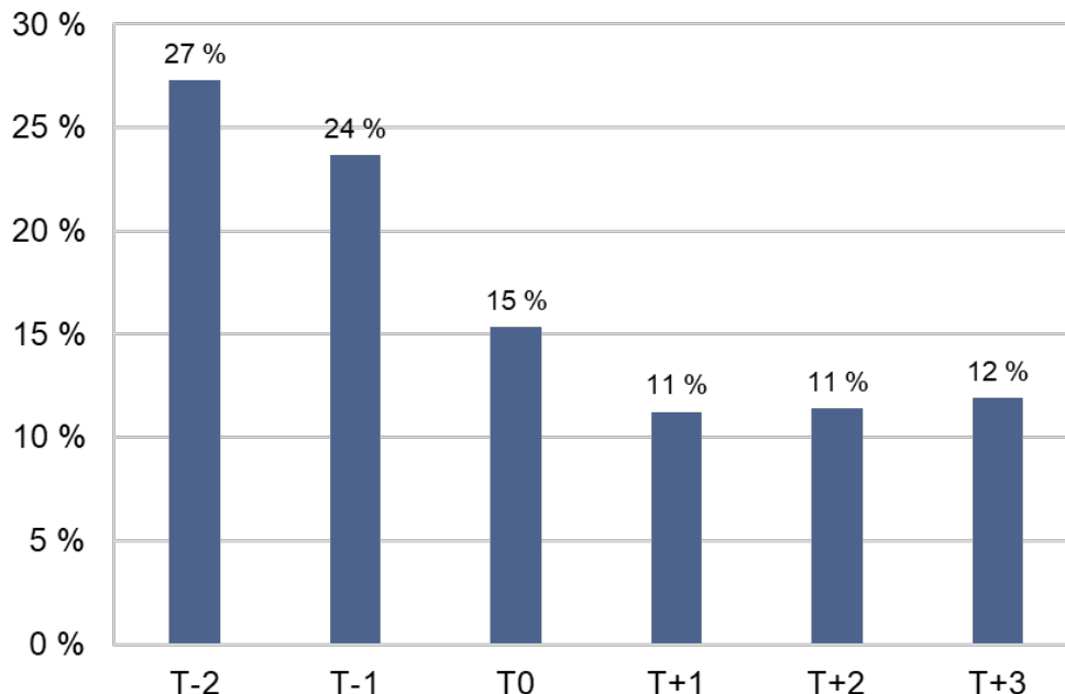
Diagram 11. Andel deltagare med registrerad arbetslöshet, från två år innan avslut till tre år efter avslut.
