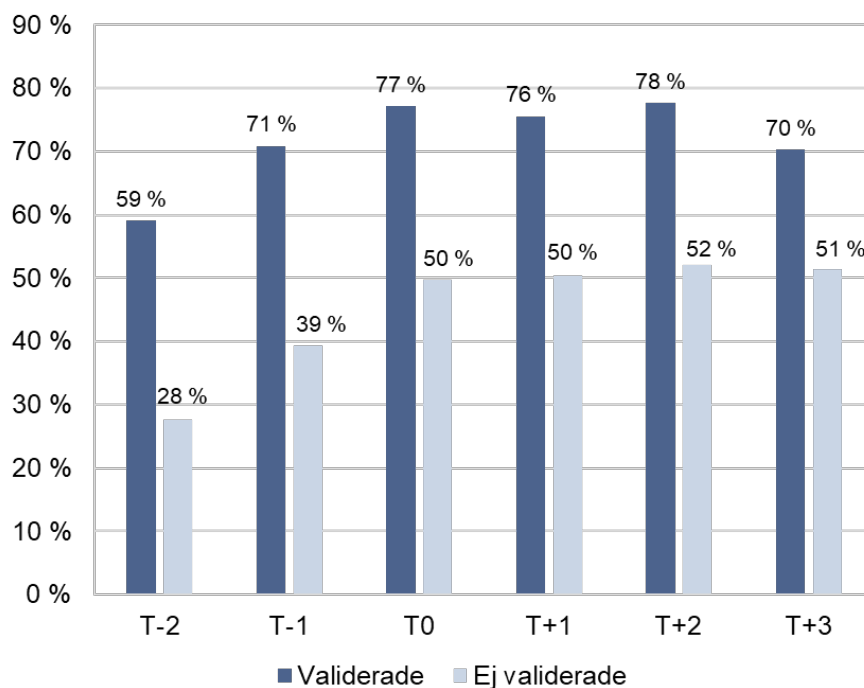
Diagram 9. Huvudsakligt arbete inom tolkbranschen, efter validerade och ej validerade, två år innan avslut till tre år efter avslut. Avser de i arbete under det aktuella året.
