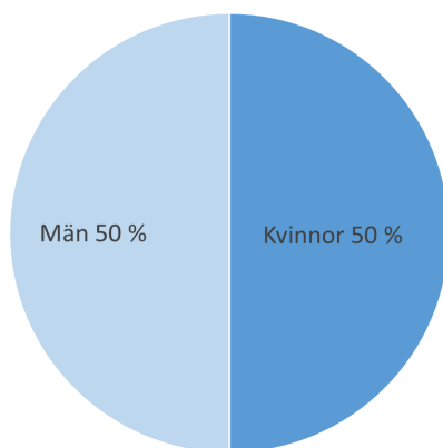
Diagram 1. Könsfördelning bland deltagarna.
